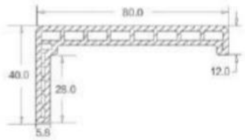
8040 木塑80×40线条 材 质：木塑(WPC) 可选木纹：任意木纹
