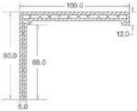
100×80 木塑100×80线条 材 质：木塑(WPC) 可选木纹：任意木纹
