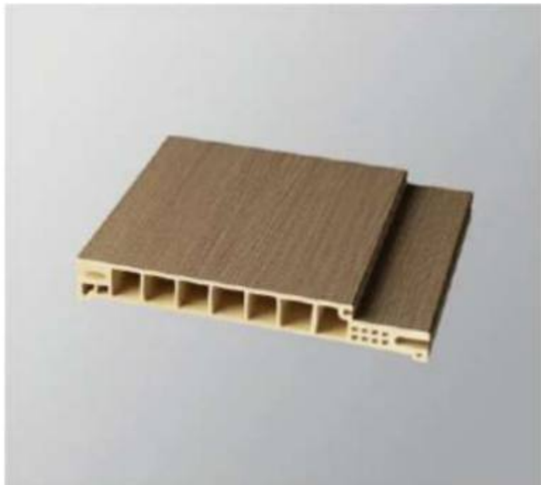
A240 A型门套240 材 质：木塑(WPC) 可选木纹：任意木纹
