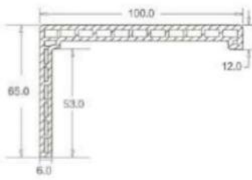
100×65 木塑100×65线条 材 质：木塑(WPC) 可选木纹：任意木纹
