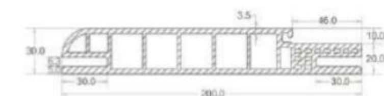
Y200 200圆弧门套 材 质：木塑(WPC) 可选木纹：任意木纹
