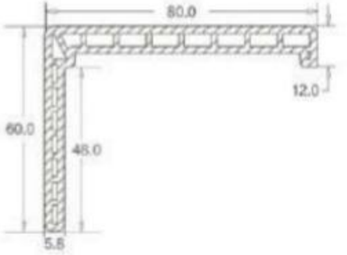
8060 木塑80×60线条 材 质：木塑(WPC) 可选木纹：任意木纹
