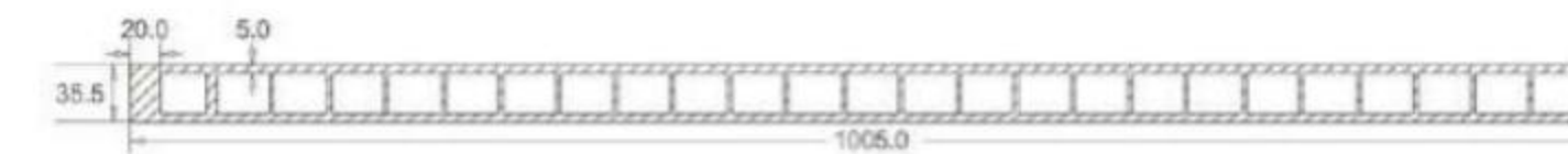
木塑门扇 35 厚 CAD
