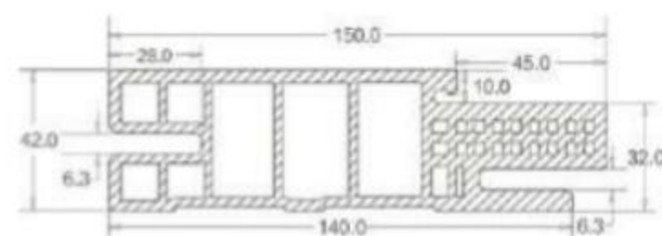
E140 E型门套E140 材 质：木塑(WPC) 可选木纹：任意木纹
